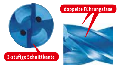
Bohrungs-Aufweitung
